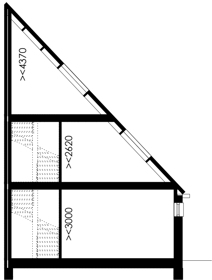
DOORSNEDE
