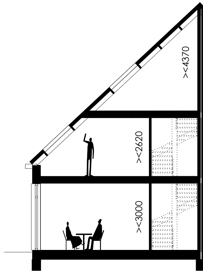
DOORSNEDE
