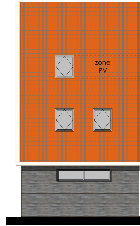
RECHTER ZIJGEVEL
